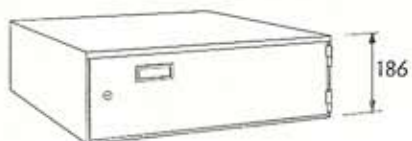
4/5 Låsbart fack. Rosengrens lås typ F 6 Inv. dim: h = 155, b = 475, d = 367 mm
