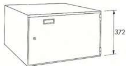
5/5 Låsbart fack. Rosengrens lås typ F 6 Inv. dim: h = 341, b = 475, d = 367 mm
