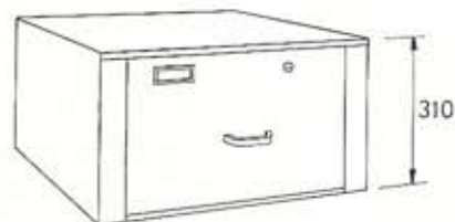
7/5 Låsbart vertikalfack för folioformat. Rosengrens lås typ F 6. Inv. dim: h = 265, b = 400, d = 352 mm Lådan kan inredas med skena för hängmap- par eller flyttbara vippstöd för stämappar.
